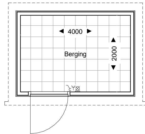
Plattegrond
