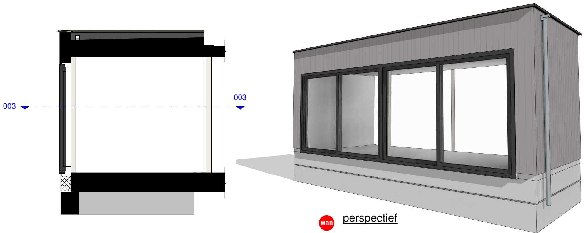
MBB 003-A 1 : 50
